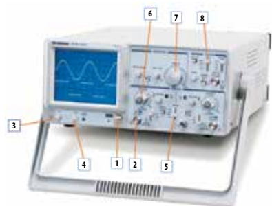
▲ Hình 1.4. Mặt trước của dao động kí
