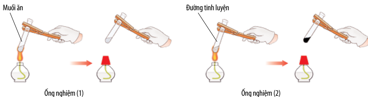
▲ Hình 6.13. Thí nghiệm so sánh khả năng bền nhiệt của muối và đường
