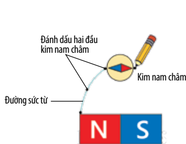
▲ Hình 19.4. Cách vẽ đường sức từ
