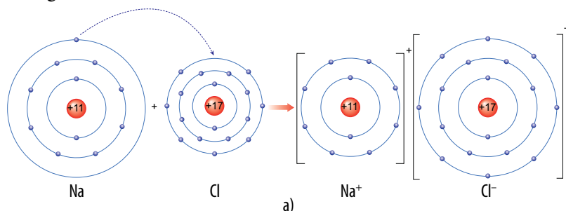
▲ Hình 6.4. a) Sơ đồ tạo thành liên kết ion trong phân tử sodium chloride b) Hình mô phỏng phân tử sodium chloride
