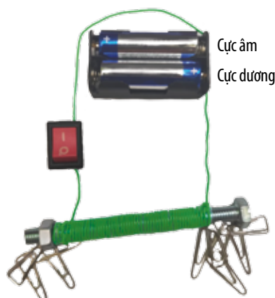
▲ Hình 21.2. Thí nghiệm tạo nam châm điện với hai pin 1,5V
