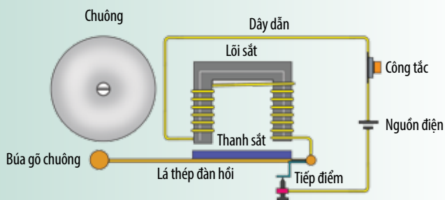
▲ Sơ đồ cấu tạo của chuông điện
