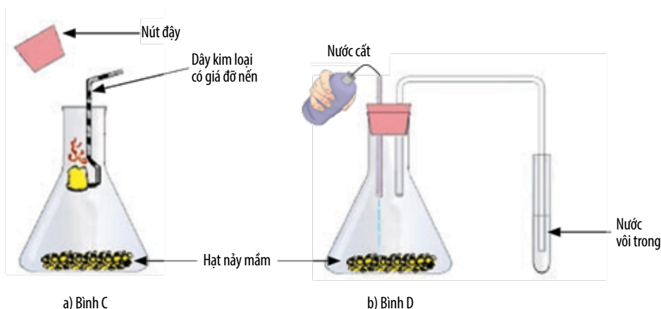
▲ Hình 26.2. Cách bố trí thí nghiệm
