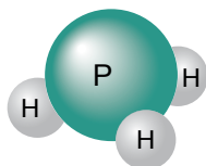
c) Phosphine
