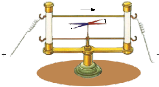
▲ Hình 19.2. Thí nghiệm Oersted
