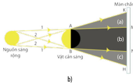
▲ Hình 15.6. a) Thí nghiệm tạo vùng tối bởi một nguồn sáng rộng; b) Hình vẽ biểu diễn vùng tối tạo bởi một nguồn sáng rộng
