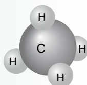
▲ Hình mô phỏng phân tử methane
