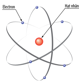
▲ Hình 2.4. Mô hình nguyên tử của Rutherford
