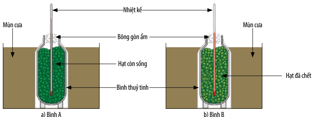
▲ Hình 26.1. Mô phỏng kết quả thí nghiệm
