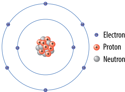
▲ Hình 2.6. Mô hình nguyên tử oxygen (O)
