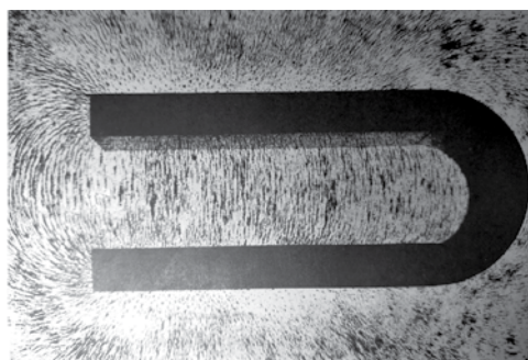
▲ Từ phổ của nam châm chữ U
