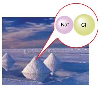
▲ Hình 5.8. Ruộng muối và hình mô phỏng phân tử muối ăn
