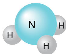
▲ Hình 5.4. Hình mô phỏng phân tử ammonia
