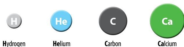
▲ Hình 3.3. Kí hiệu hoá học của một số nguyên tố
