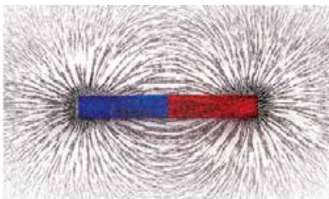
▲ Hình 19.3. Từ phổ của thanh nam châm
