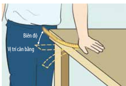
▲ Hình 13.1. Biên độ dao động của thước
