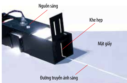
▲ Hình 15.3. Tạo chùm sáng hẹp song song
