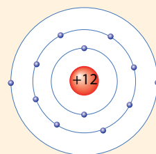
▲ Mô hình nguyên tử magnesium (Mg)
