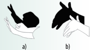
▲ Tạo bóng các con vật trên tường
