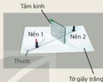
Hình 17.2 Bố trí thí nghiệm kiểm tra tính chất ảnh của vật qua tấm kính
