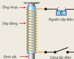
Hình 20.2 Sơ đồ cấu tạo nam châm điện đơn giản
