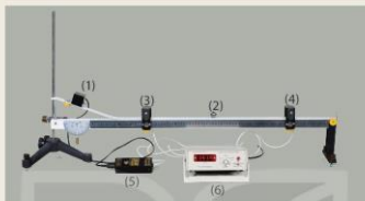
Hình 9.3 Thí nghiệm đo tốc độ bằng đồng hồ hiện số và cổng quang
