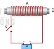
Hình 20.1 Cấu tạo của nam châm điện
