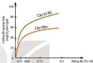
Hình 23.2 Biểu đồ thể hiện ảnh hưởng của nồng độ khí \text{CO}_2 ngoài môi trường đến quang hợp ở cây bí đỏ và cây đậu*
