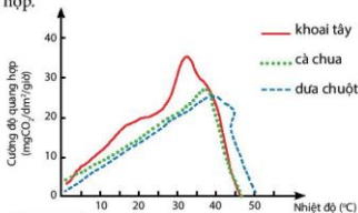
Hình 23.3 Biểu đồ thể hiện ảnh hưởng của nhiệt độ đến quang hợp ở cây khoai tây, cây cà chua và cây dưa chuột*
