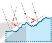
Hình 16.4 Phản xạ khuếch tán
