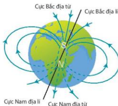
Hình 19.7 Mô phỏng từ trường Trái Đất
